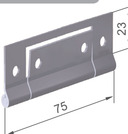
Scharnier 40 kg
