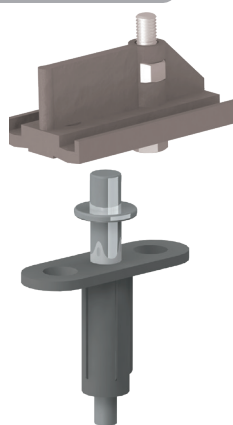
oberer Drehzapfen mit Aufnehmer
