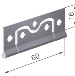
Scharnier 25 kg
