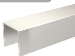
U-Profil verzinkt Maße 25x17 mm, Länge 2000 mm
